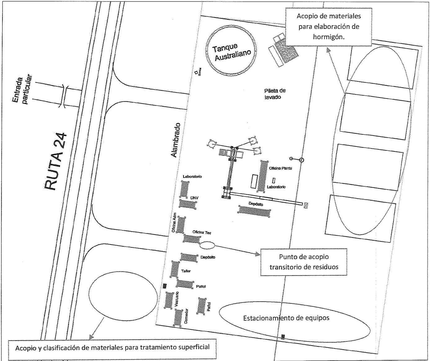
Croquis del campamento de "Nueva Mehlem" ubicado en el km. 28,5 de la ruta 24. Se destaca la ubicación de los acopios de materiales granulares.
